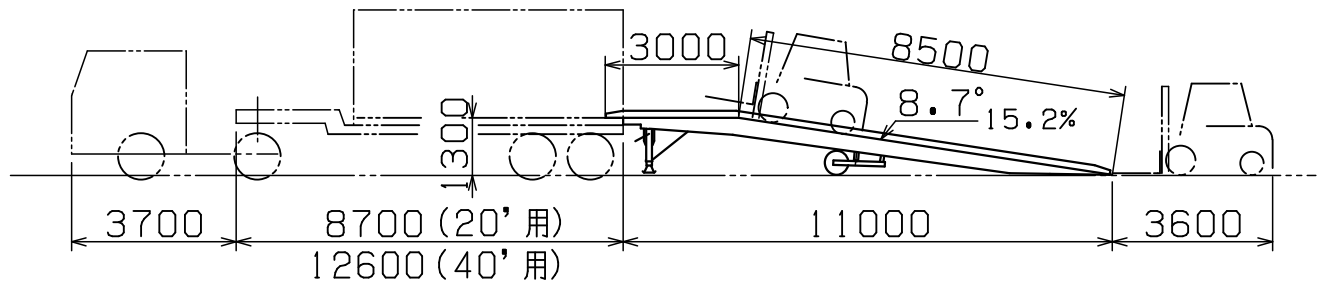
全体配置図 (例)
