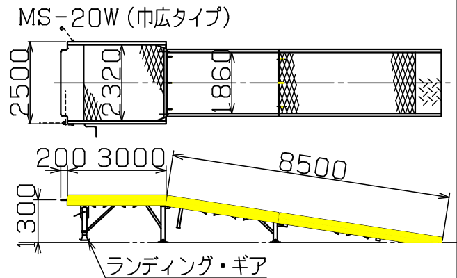
ランディングブリッジ (分割型、簡易式)
