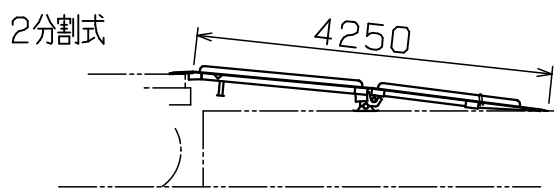
プラットフォーム上スロープ
