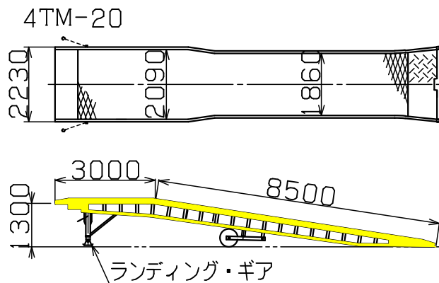
ランディングラン (一体型、油圧昇降式)
