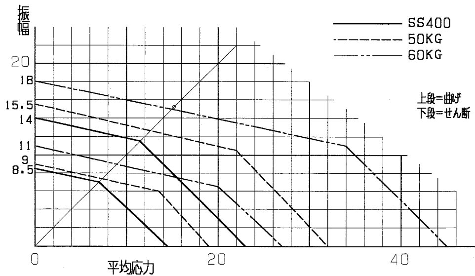
母材の限度線図
