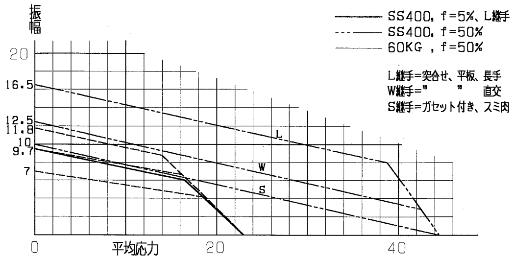
溶接継手の限度線図
